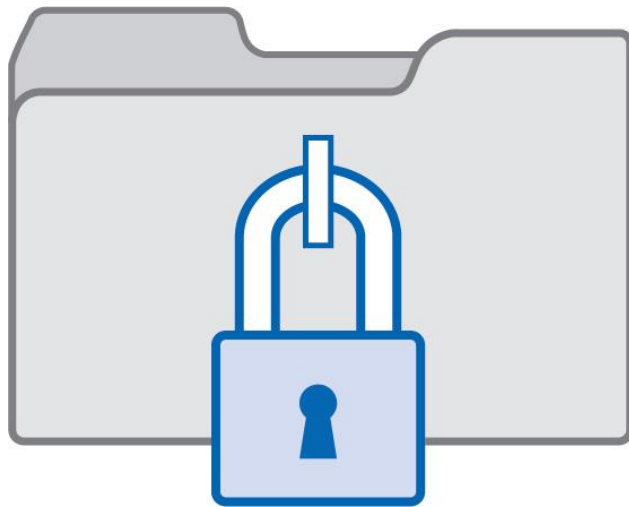
Доменная аутентификация
