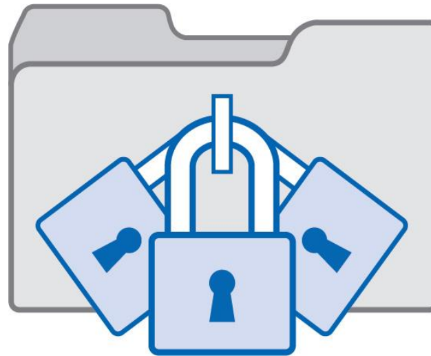
Многофакторная аутентификация
